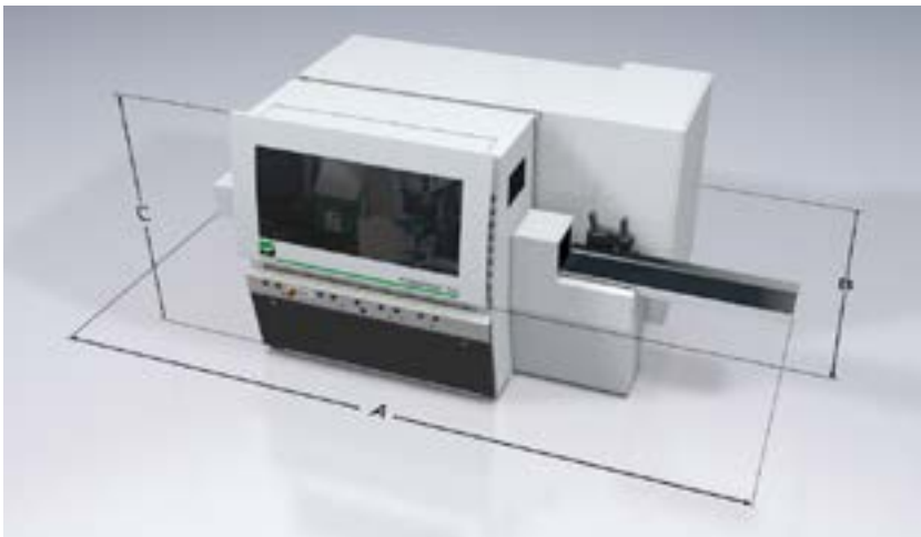
017 A = 3820 mm, B = 1805 - 2155 mm, C = 1900 mm
